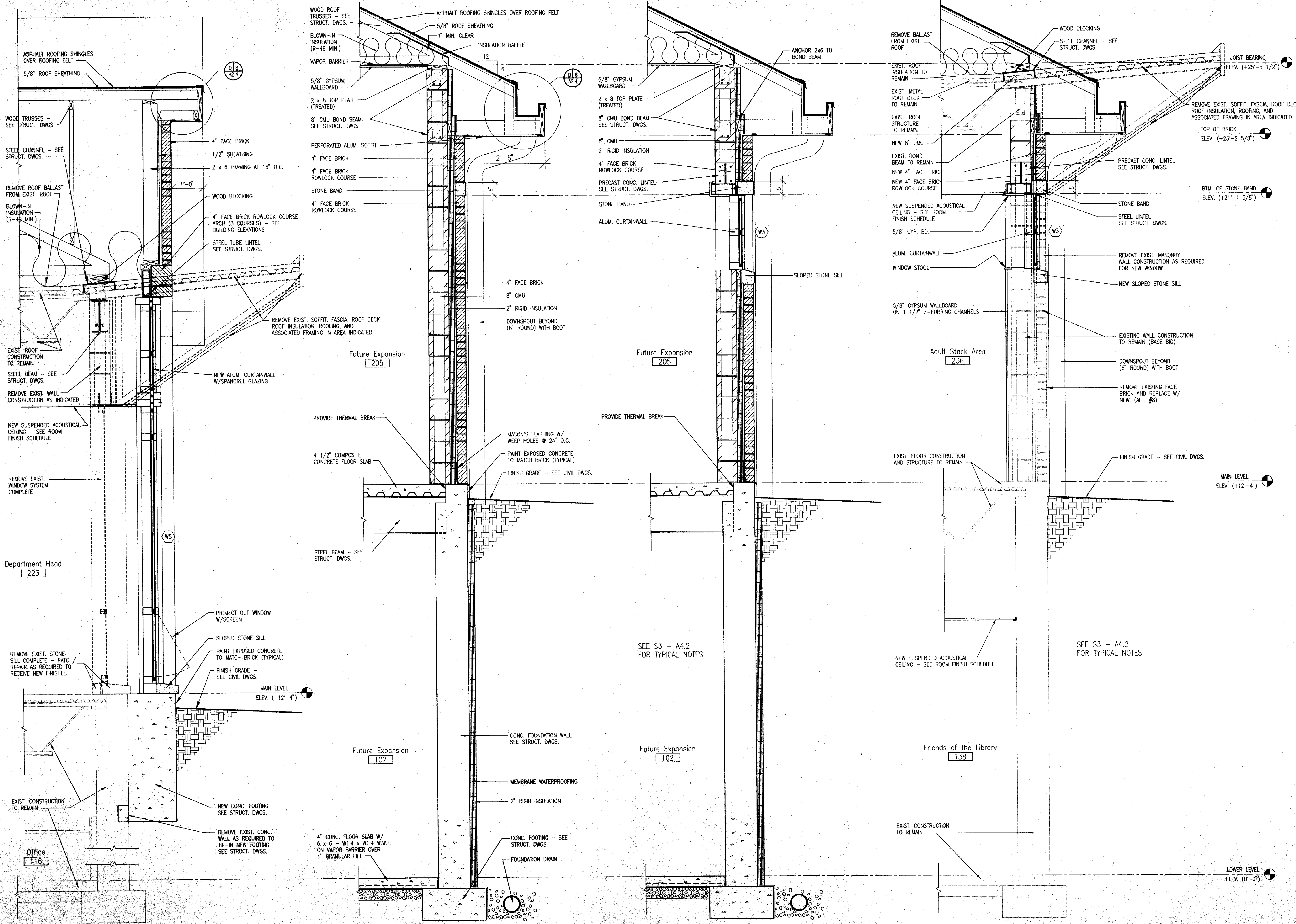
WALL SECTION S4 SCALE: 3/4" = 1'-0"
